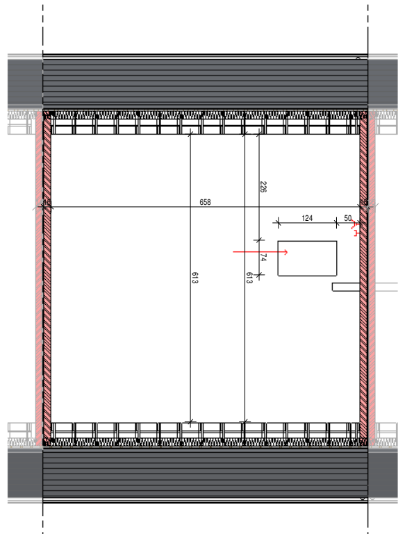
2de verdieping
