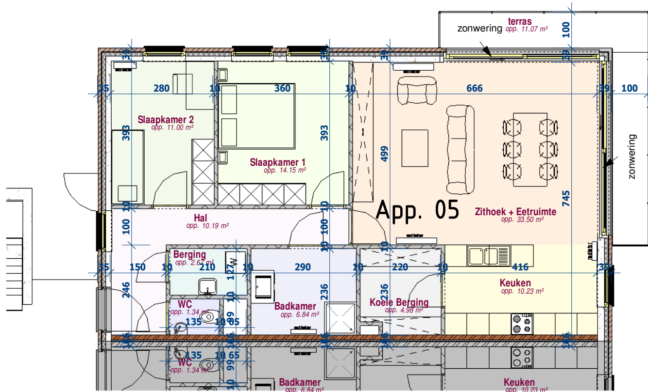
1 App. 05 1 : 100
