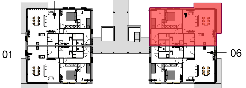
1 App. 05 - situering 1 : 400
