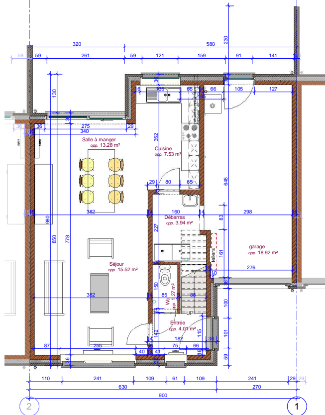
1 Rez-de-chaussée - lots 07-08 et 09-10 1 : 50
