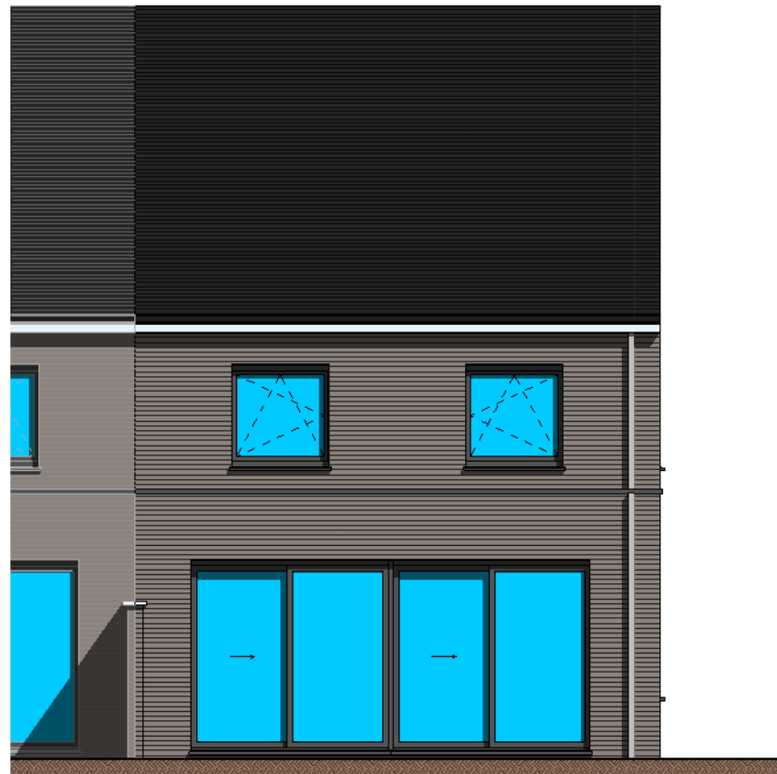
1 ACHTERGEVEL 1 : 50
