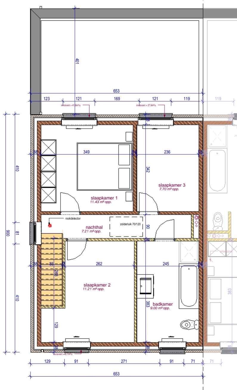
2 1ste VERDIEPING 1 : 50
