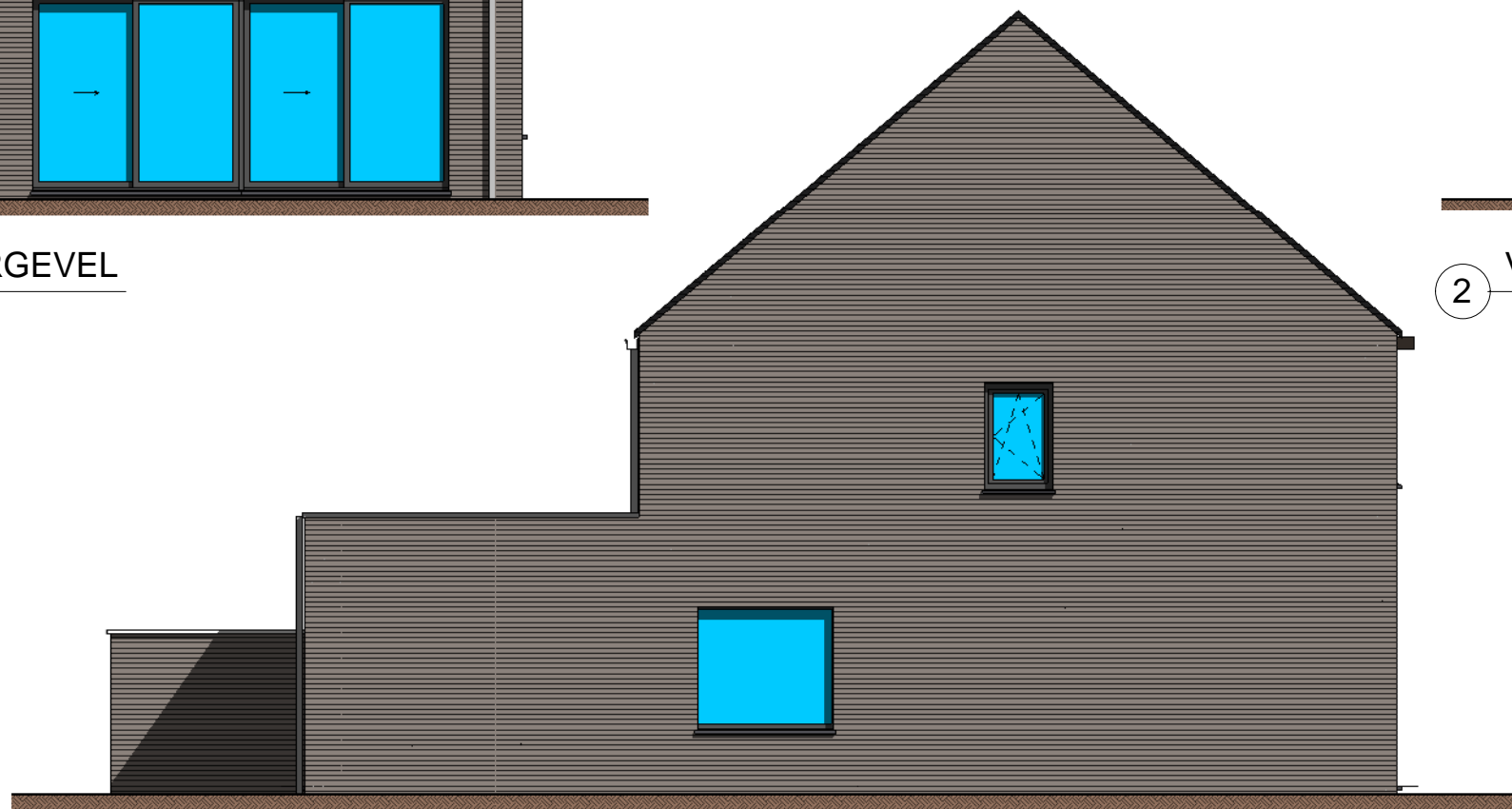
3 ZIJGEVEL LINKS 1 : 50
