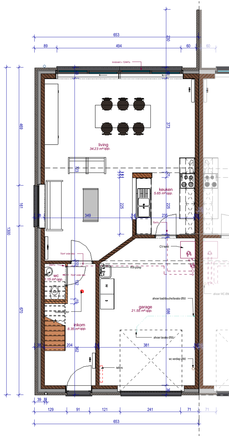
1 GELIJKVLOERS 1 : 50
