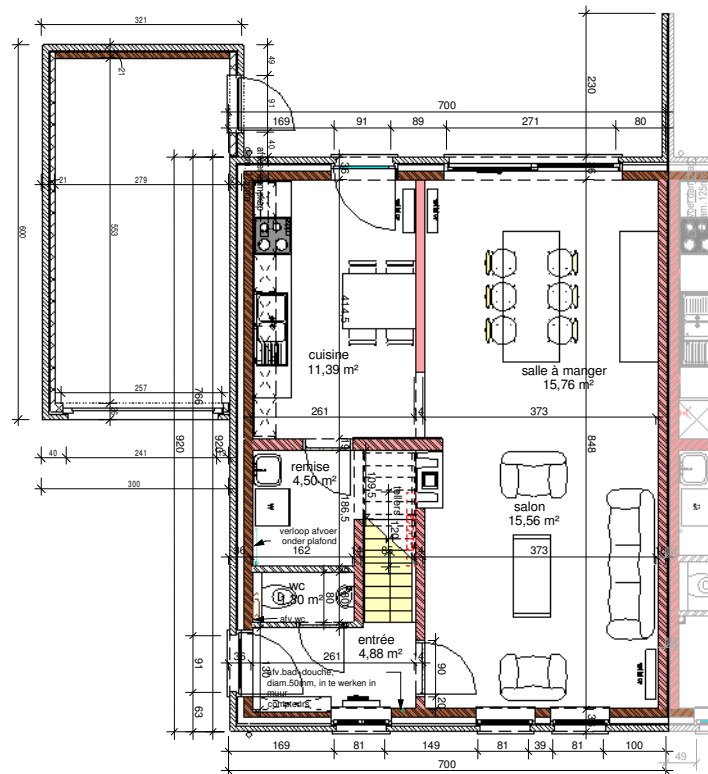
1 rez-de-chaussee 1 : 50
