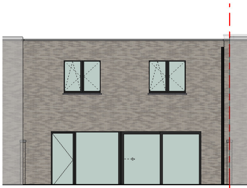
lot 120 achtergevel
