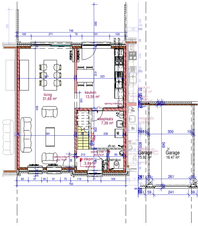
gelijkvloers
