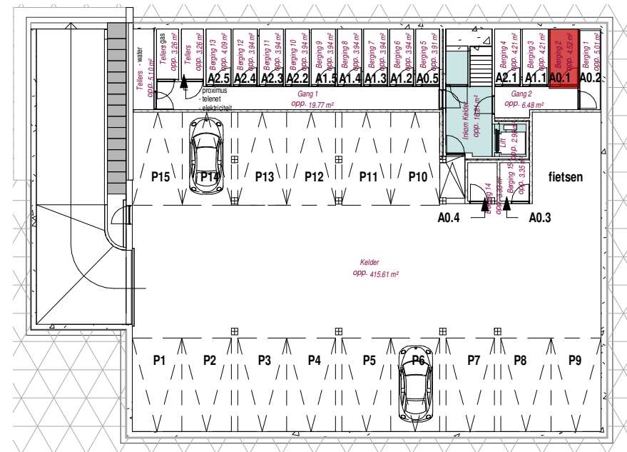
berging 0.1
