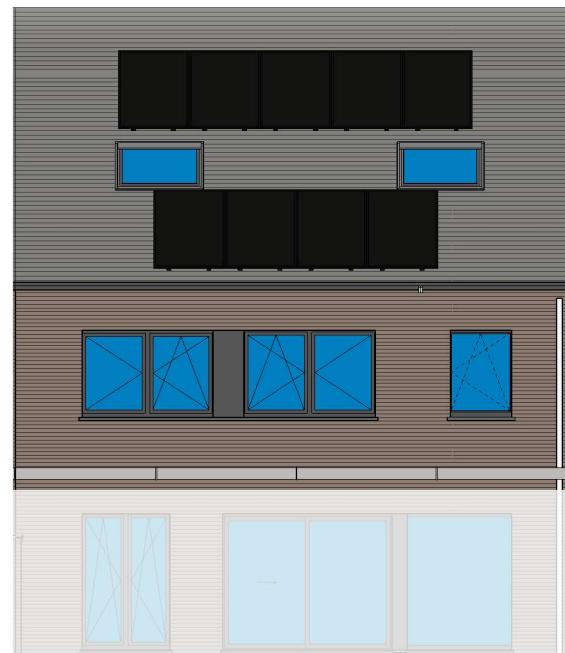
achtergevel lot 13b LL
