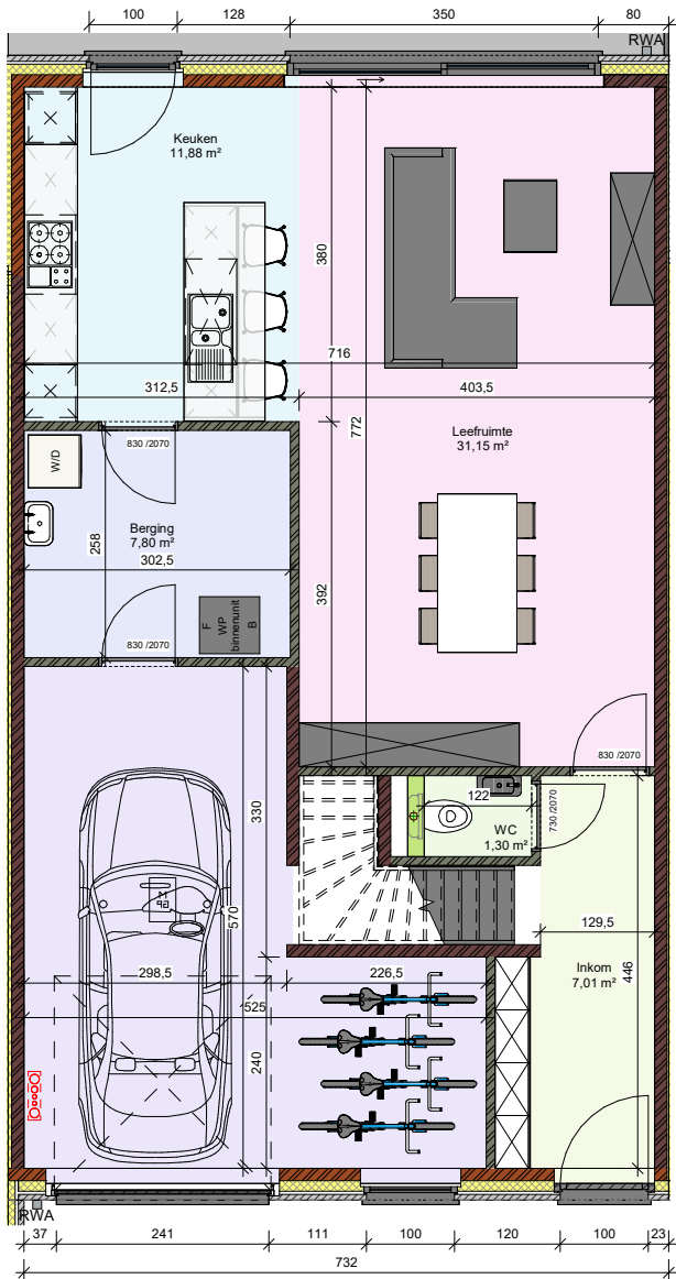
Gelijkvloers LL - lot 2
