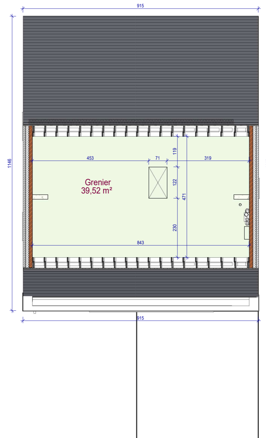
2e étage lot 31
