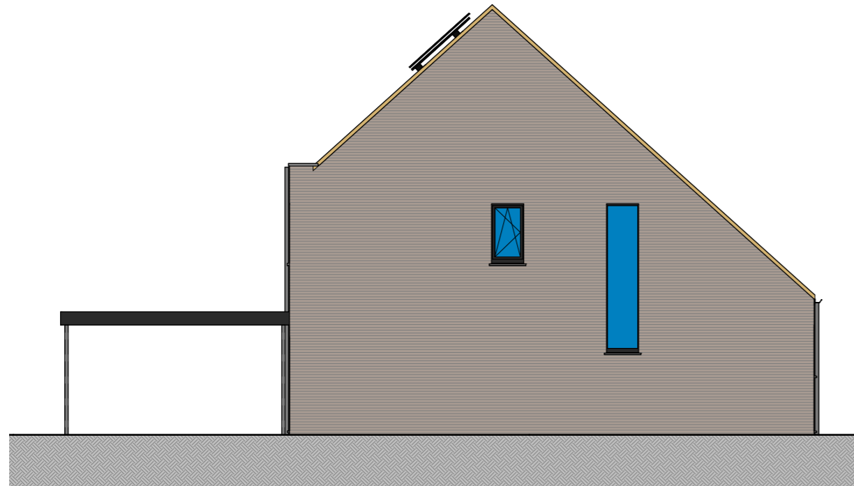
Façade laterale droite lot 31
