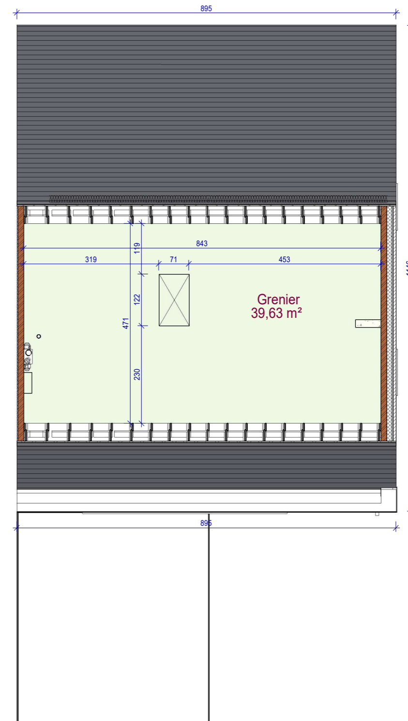
2e étage lot 38
