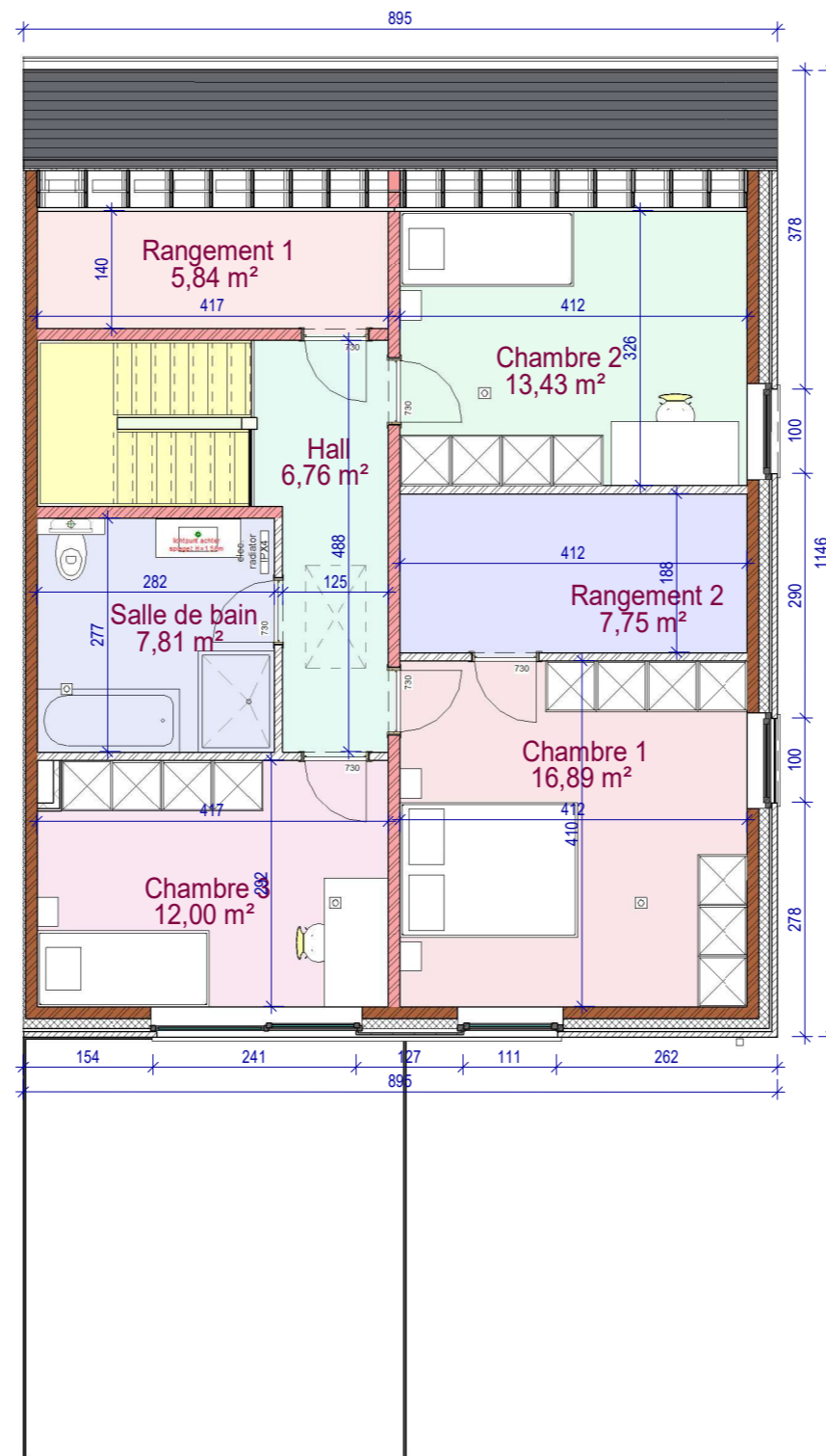
étage lot 40
