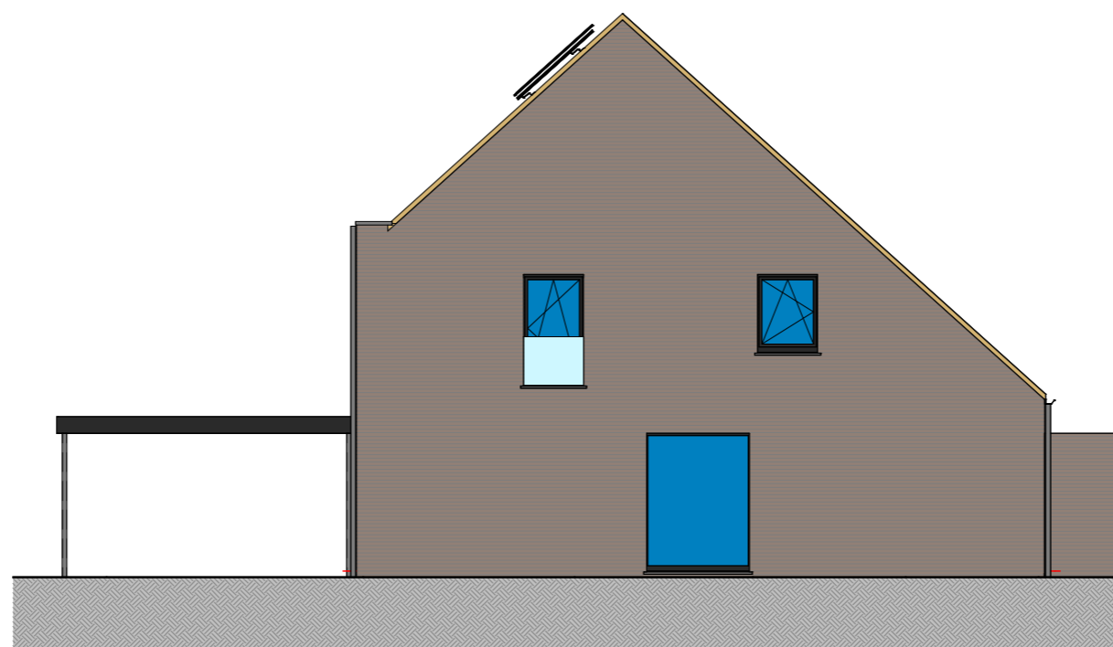
Façade laterale droite lot 40
