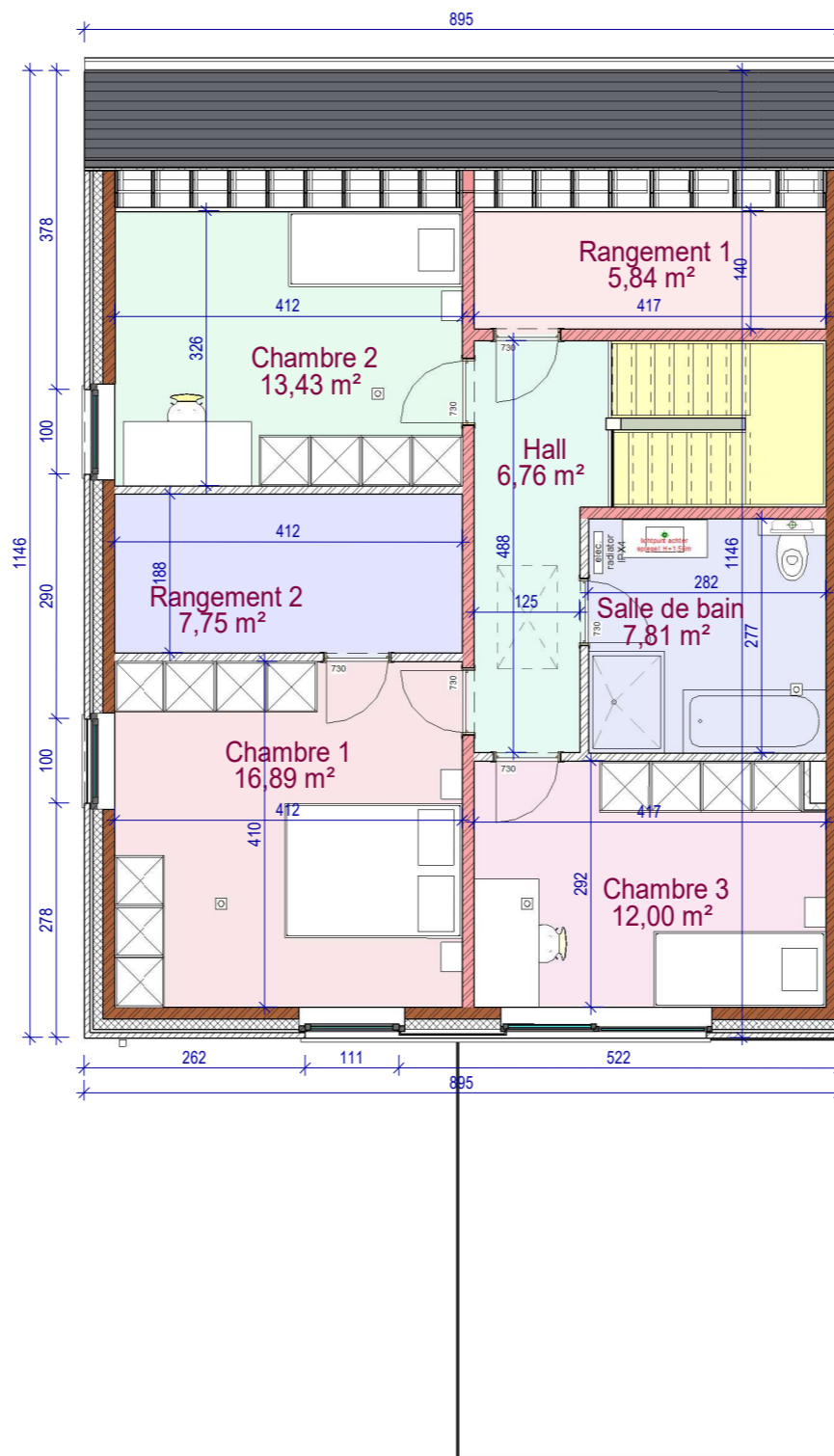
étage lot 41
