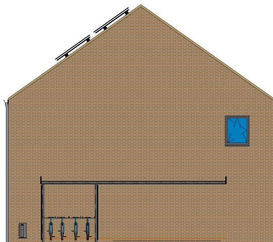
Zijgevel links
