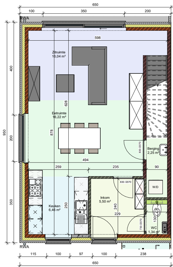
Gelijkvloers LL - lot 7
