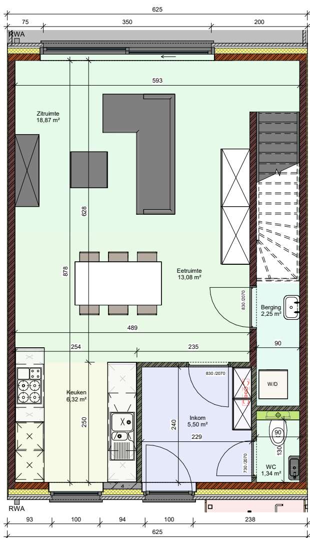
Gelijkvloers LL - lot 9
