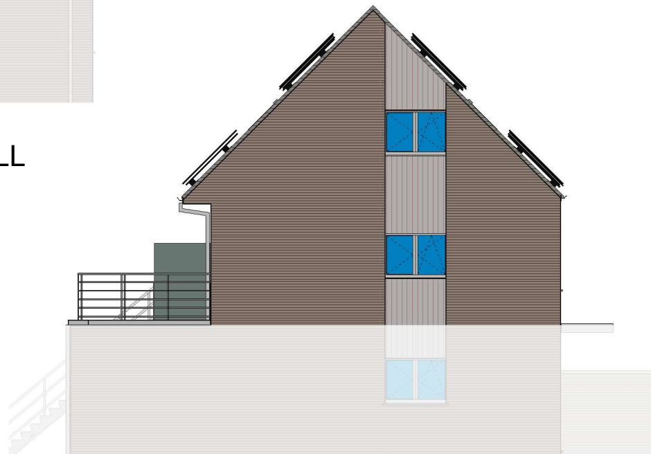
zijgevel rechts lot 9b LL
