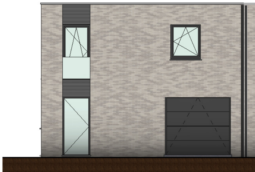
voorgevel
