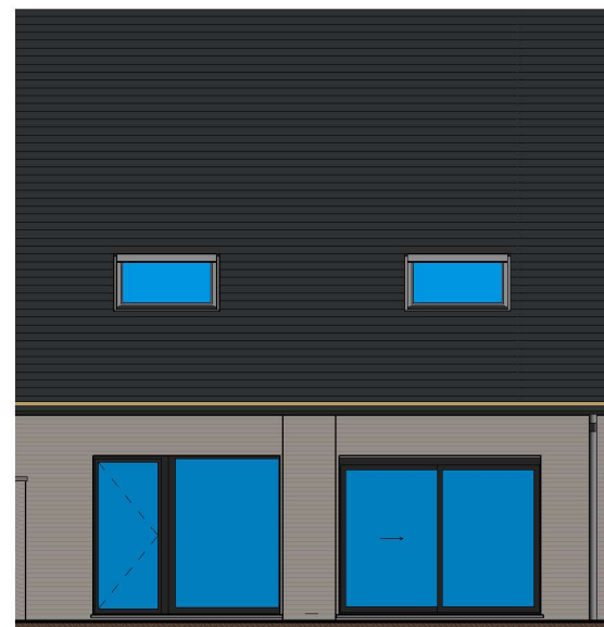
2 Achtergevel lot 216 LL 1 : 70
