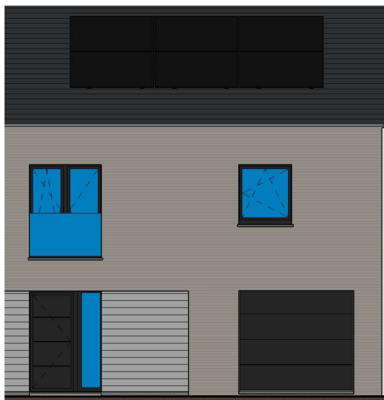
1 Voorgevel lot 216 LL 1 : 70
