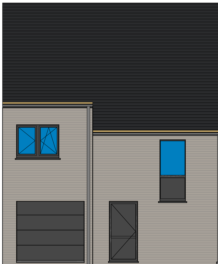
2 voorgevel woning 2 1 : 75
