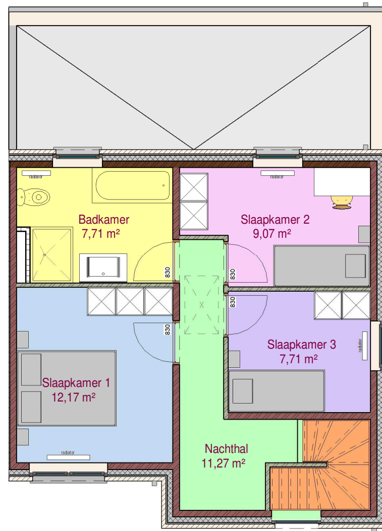
2 verdieping woning 2 LL 1 : 75
