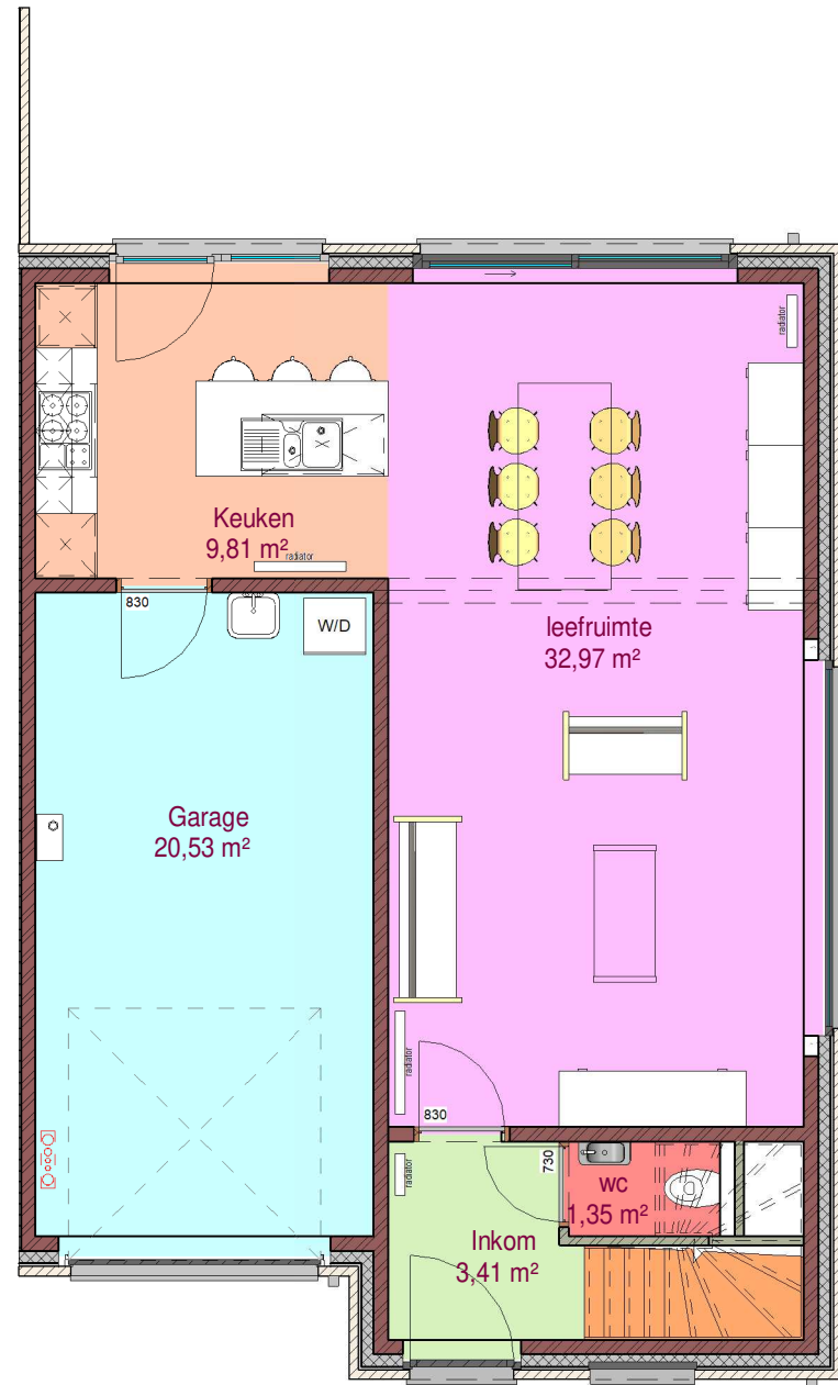
1 gelijkvloers woning 2 LL 1 : 75
