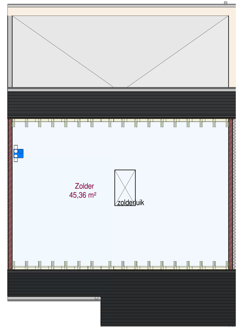
3 2e verdieping woning 2 LL 1 : 75
