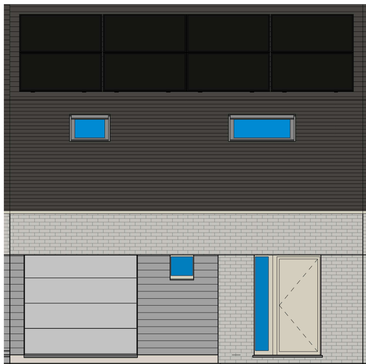
Voorgevel lot 2 LL
