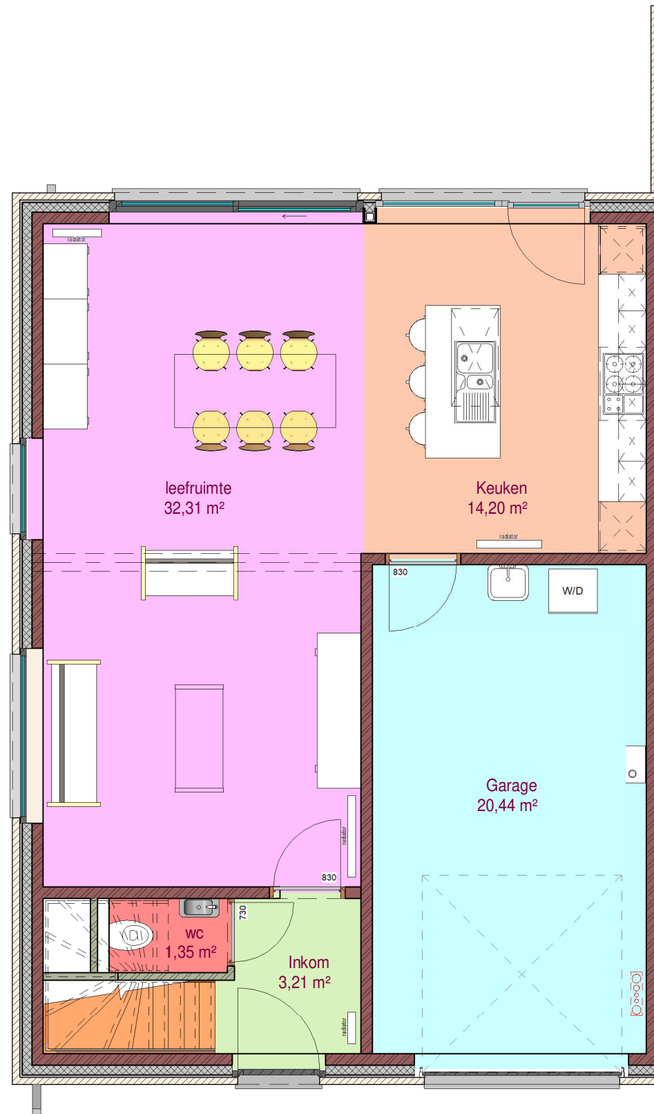
1 gelijkvloers woning 3 LL 1 : 60
