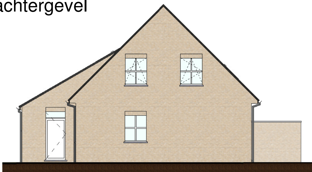
gevel rechts
