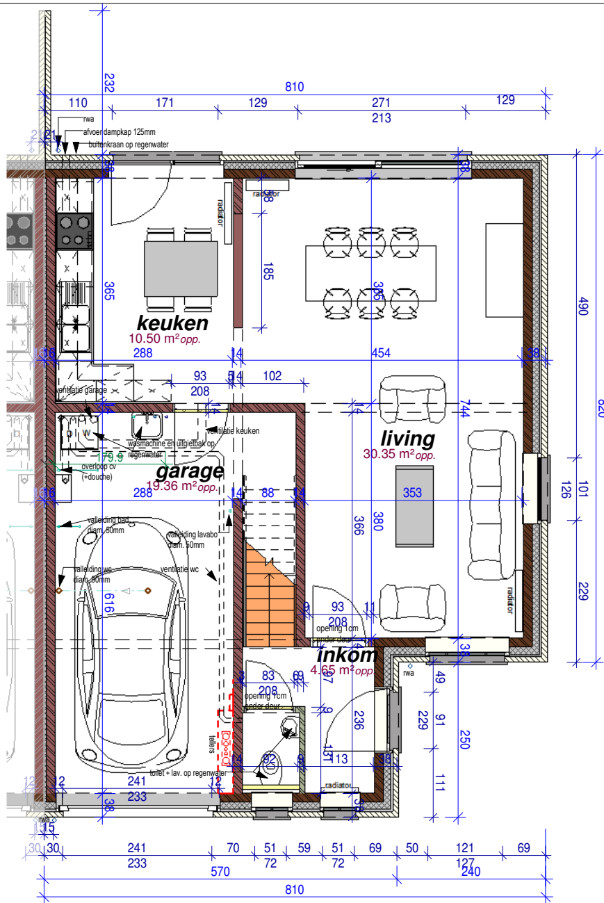
gelijkvloers
