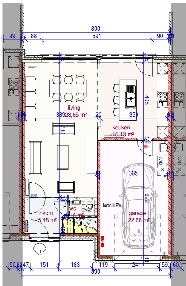
gelijkvloers
