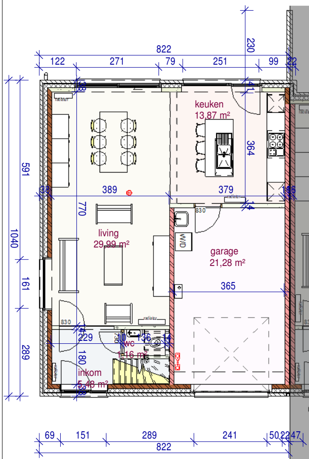
gelijkvloers
