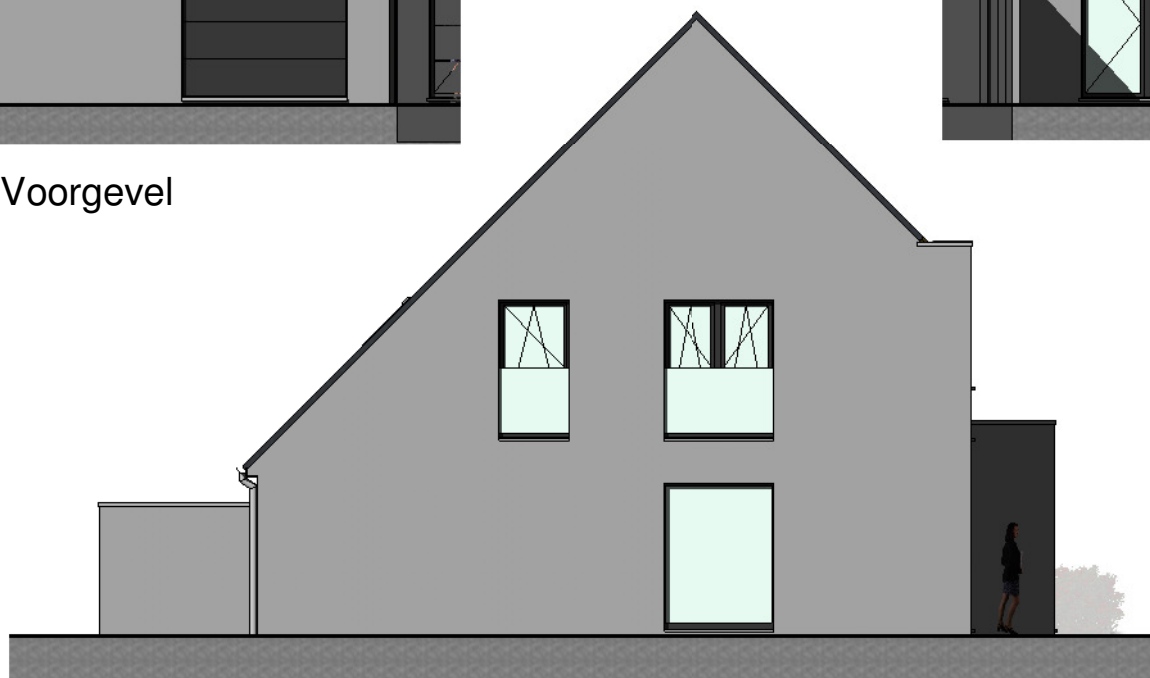
Zijgevel
