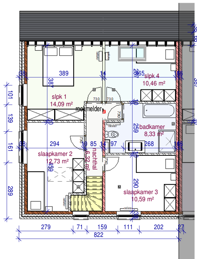
1ste verdieping
